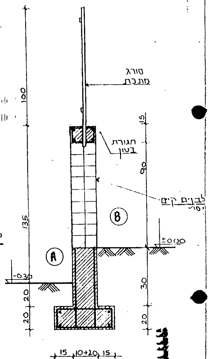
פרט גדר קנה 1:20
