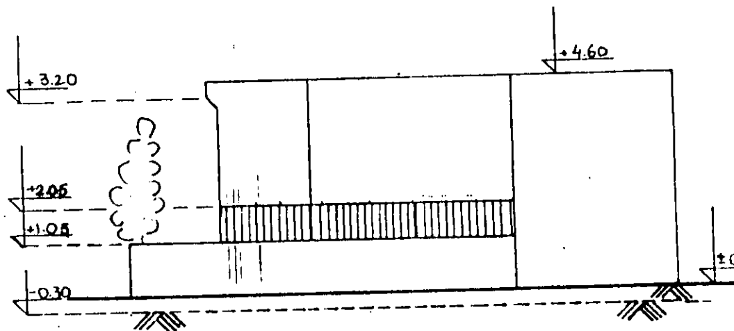
חזית דרומית קנה 1:100
